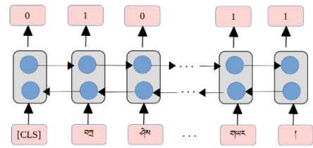
图 1 BiLSTM 的结构
