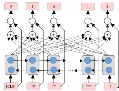
图 2 BiLSTM-Atten 的结构
